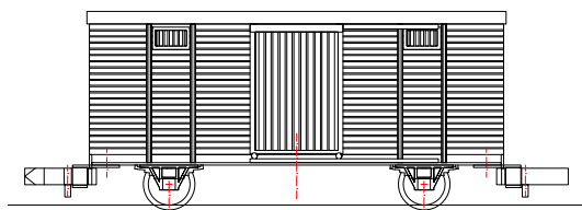
FrBB G 151 / G 152 / G 153
