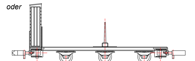
OH3 als H3 mit Bremserhaus H3 97-63-06 Netz Burg
