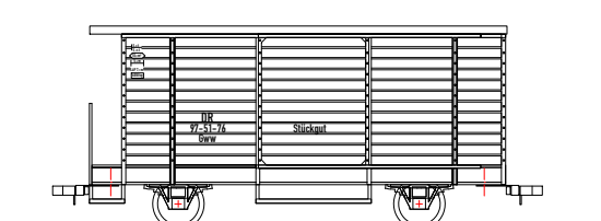
Gww 97-51-76 "Stückgut" (ex. Pollo) Gww 97-51-87 "Stückgut" Gww 97-51-77
