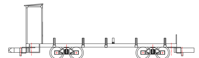
RRw 97-55-01 (Hbr.) - Stangenwagen
