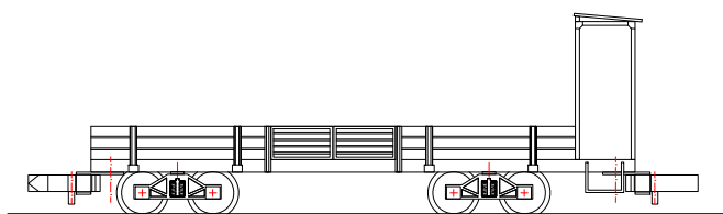
OOw 97-55-09 (Türen + Hbr.)
