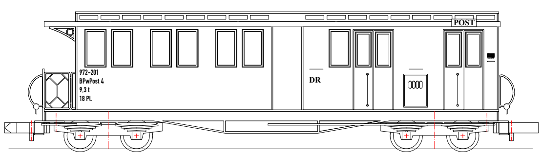
TB 1 BPwPost 4 Erf 7.0761 BPwPost 4 972-201
