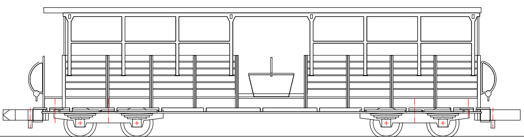
TB 30 / 31 als Sommerwagen B4tro Erf 7.1356 / 7.1357
