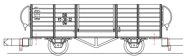
TB 41 Ow Erf 7.4241 Ow 97-38-32
