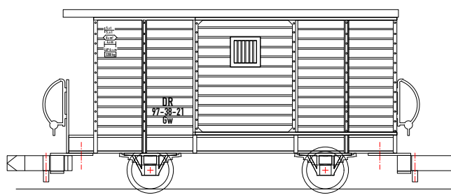
TB 20 Gw Erf 7.2221 Gw 97-38-21
