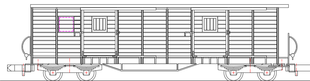
TB 10 als GGw GGw Erf 7.0763
