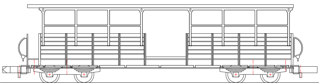
TB 30 / 31 als Stückgutwagen B4tro Erf 7.1356 / 7.1357
