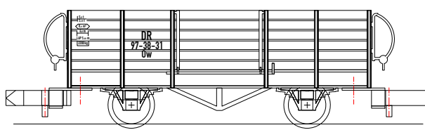
TB 40 Ow Erf 7.4240 Ow 97-38-31
