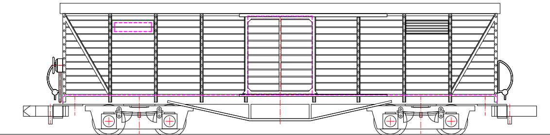
Leichtbauwagen WUMAG 1942 GGm K3527 Dre (1942) > Dre 7.3527
