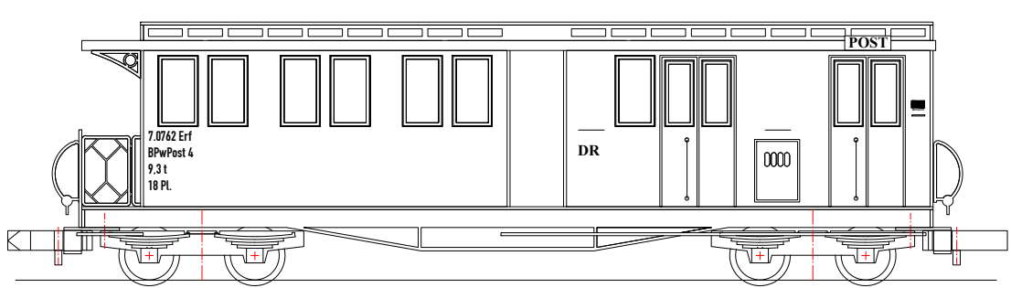
TB 2 BPwPost 4 Erf 7.0762
