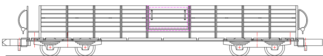
TB 30 / 31 als offener Güterwagen
