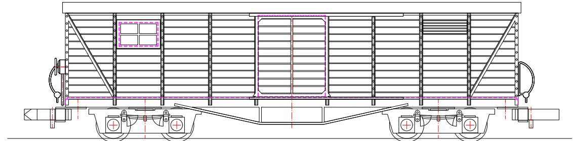
Umbau in Gerätewagen 97-38-11 (1953)
