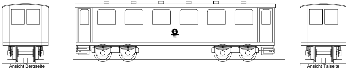
Bauart Zugspitzbahn
