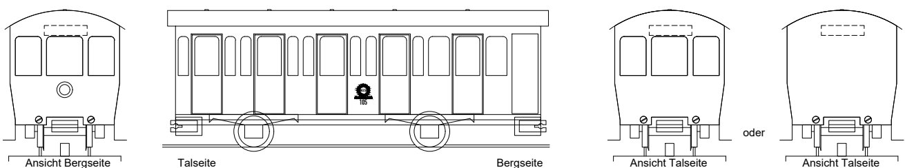
Bauart Wendelsteinbahn
